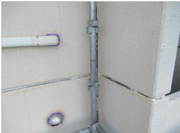
シーリング 撤去
