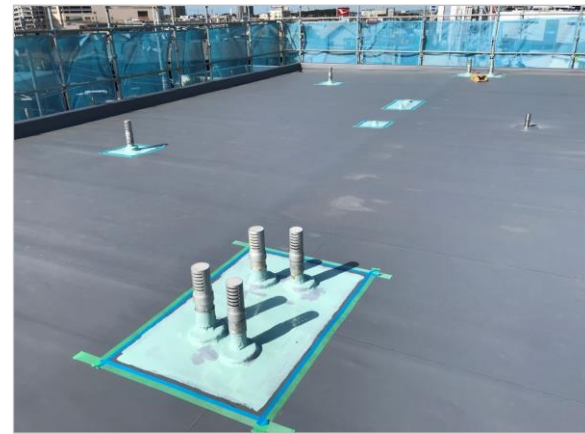
脱気筒・換気口廻り ウレタン防水工事
